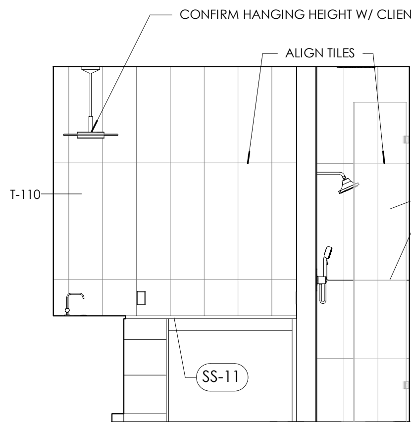
6 GUEST BATH 3 E 3/8" = 1'-0"
