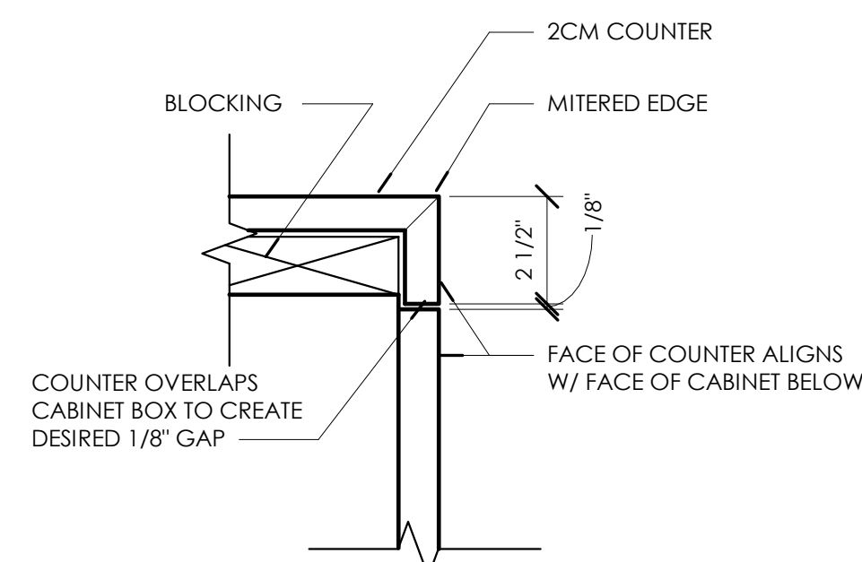
5 COUNTERTOP EDGE DETAIL 3" = 1'-0"
