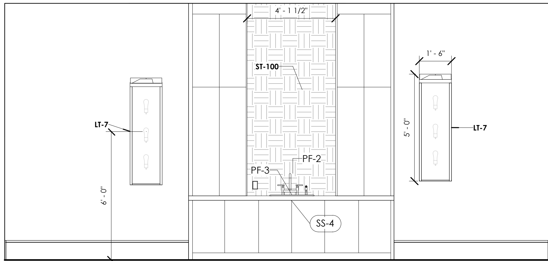
1 WET BAR 3/8" = 1'-0"
