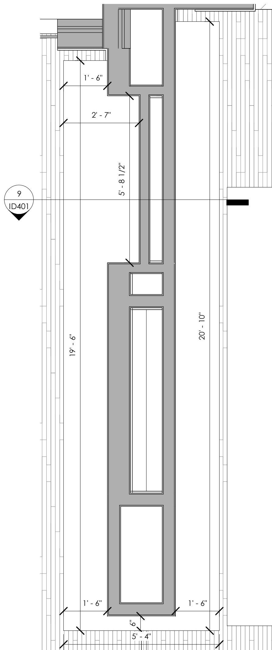
8 FIREPLACE LIVE EDGE 1/2" = 1'-0"
