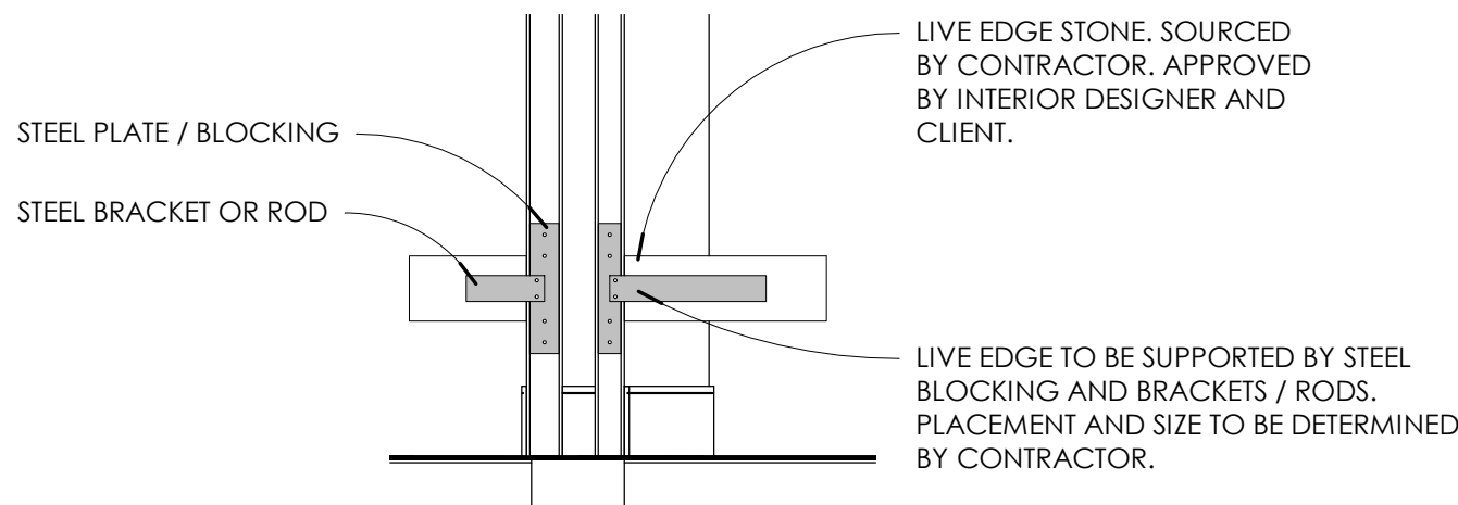
9 LIVE EDGE STONE LEDGE 3/8" = 1'-0"
